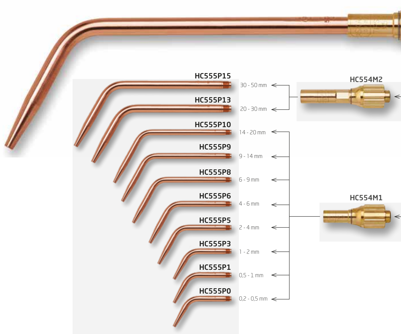
Oksi-Propan/Doğalgaz (LPG) Kaynak ve Sert Lehimleme Lüleleri Ağız Detayı
